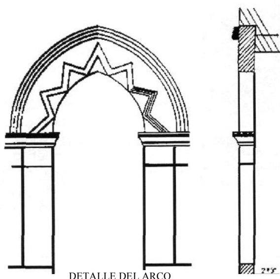
DETALLE DEL ARCO
